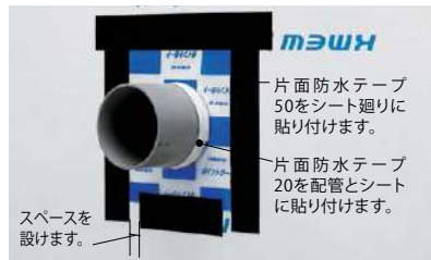
施工手順② 防水テープ貼付
