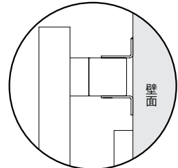
〈断面図〉
