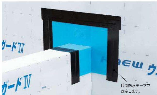
取付けイメージ バルコニー端部用
