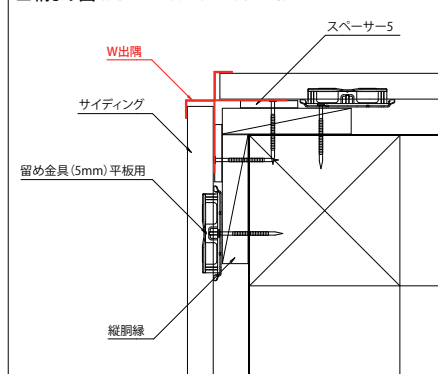
■納まり図 (横張り金具留め(5mm)施工時)
